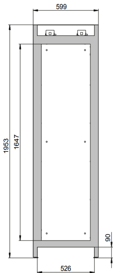
Frontalansicht
