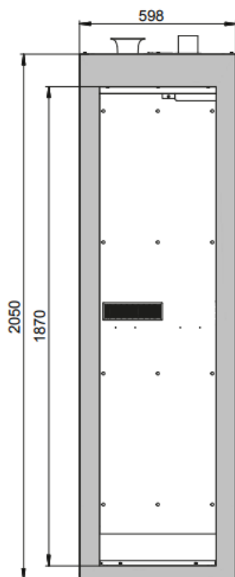
Frontalansicht
